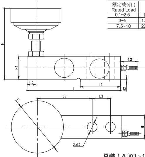
总装 (A) 0.1~10t活动压头附件
